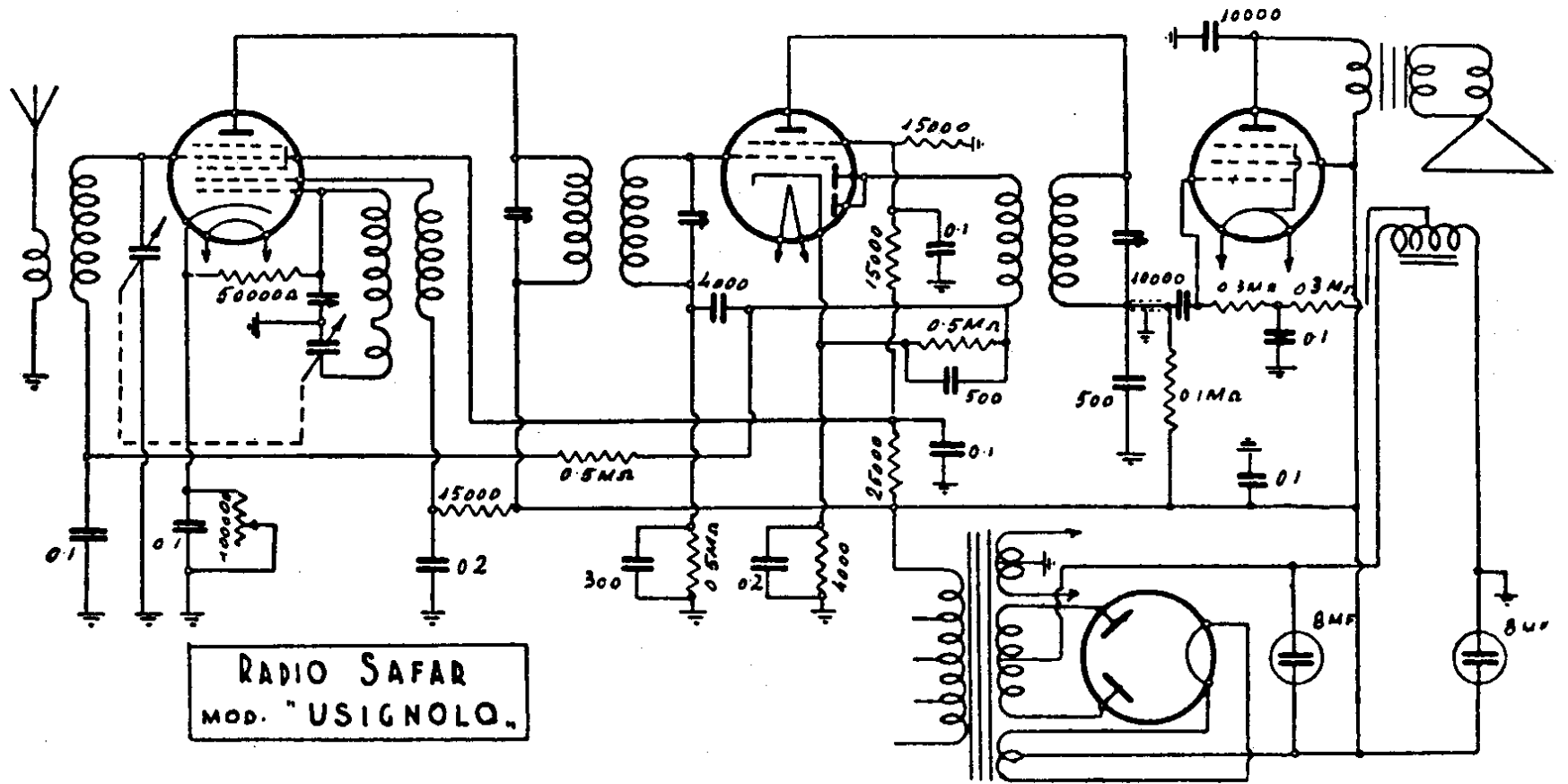
RADIO SAFAR. — Modello « Usignolo ». - Produzione 1934
